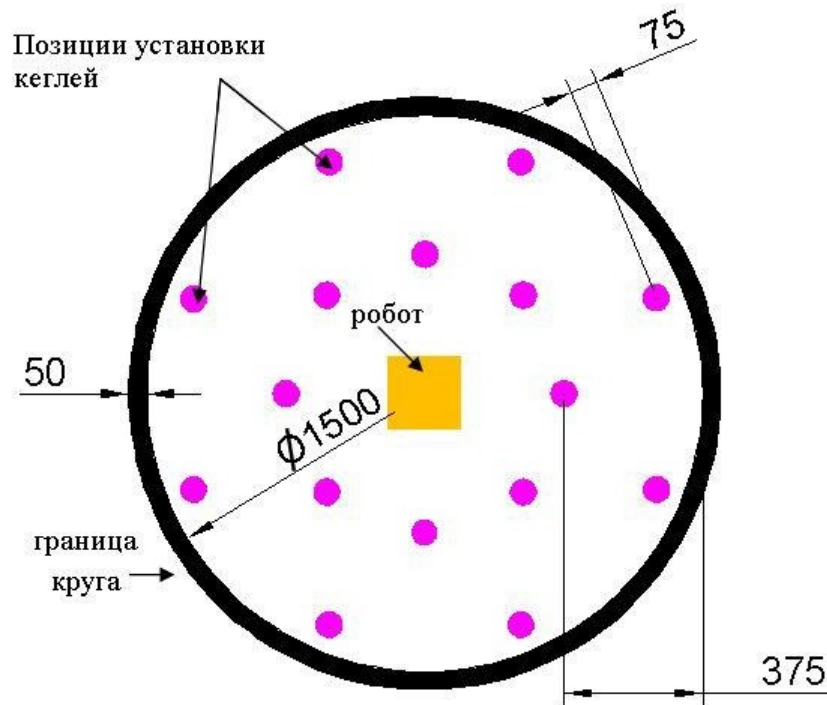
Рисунок 1 – Трасса Кегельринг макро
