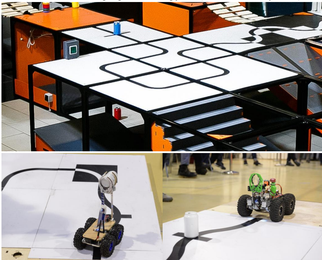
Рисунок 44 «Участки с линией (черная на белом)»
