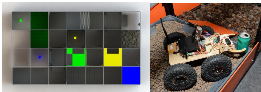
Рисунок 38 «Пример расположения маяков и зон в лабиринте»
