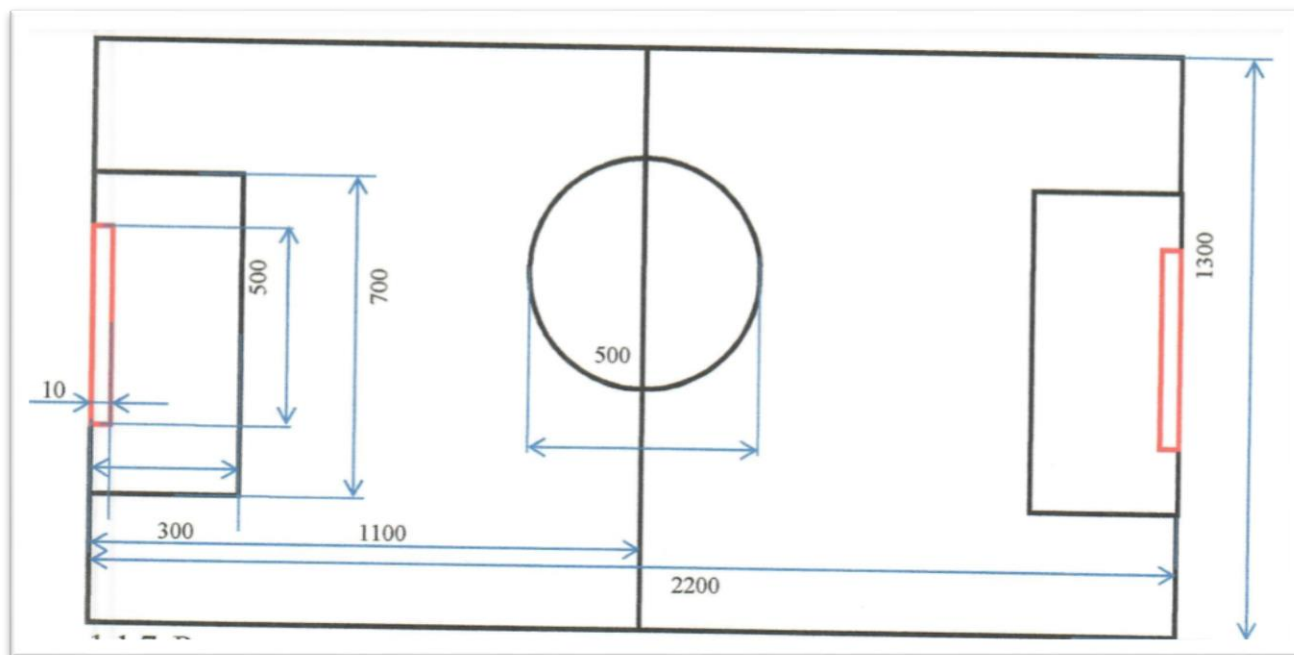
Рисунок 1 – Игровое поле
