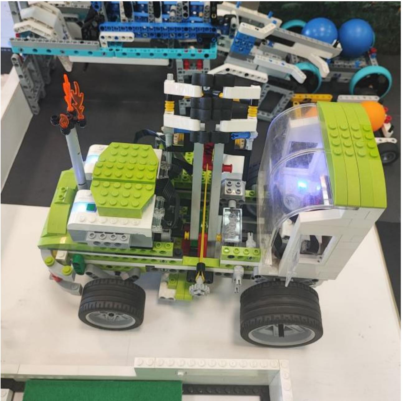
Рис. 1 Внешний вид робота-трактора «Паша»
