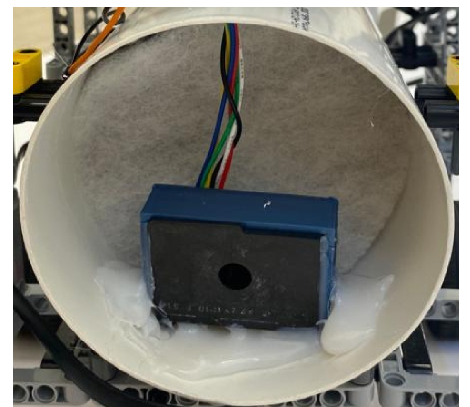
Датчик пыли и фильтр грубой очистки
