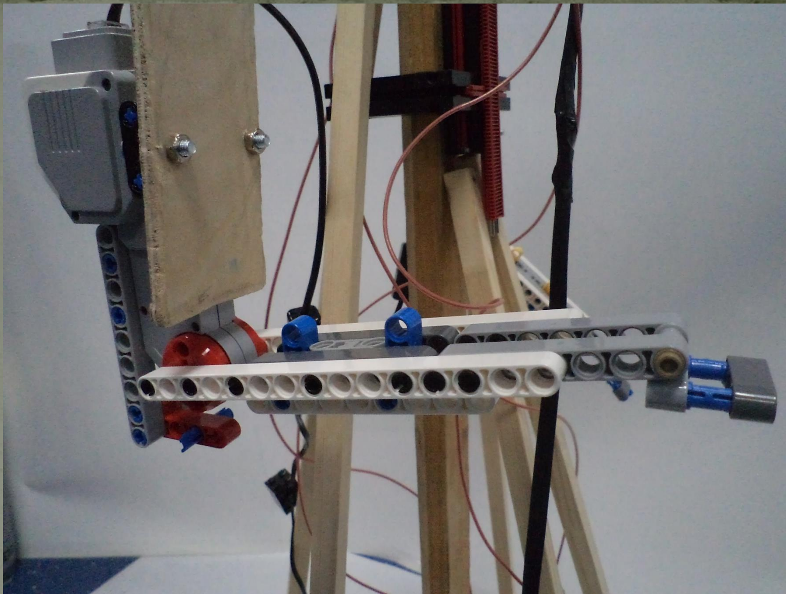
Подробная конструкция руки промотора
